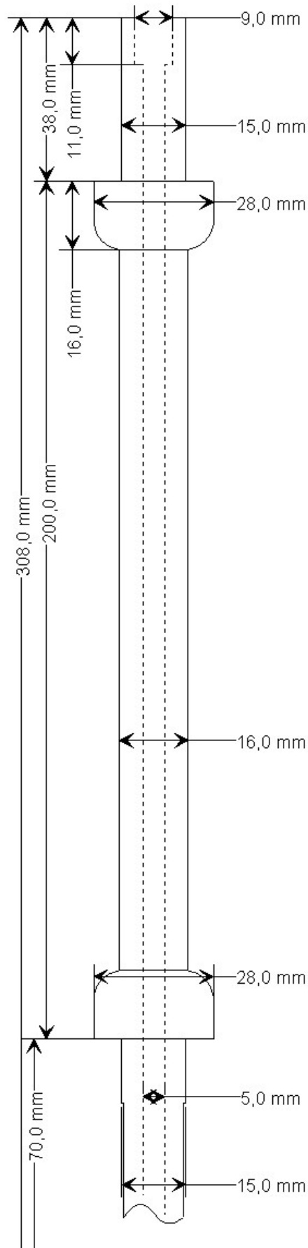
Großer Bordun - Unterteil
