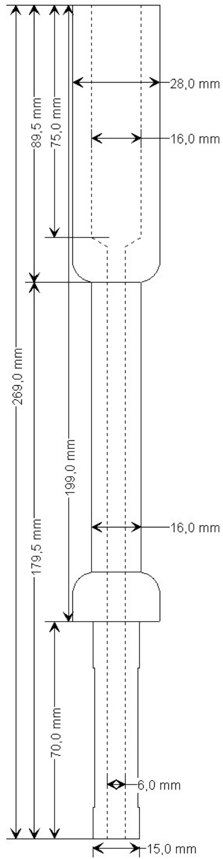
Großer Bordun - Mittelteil
